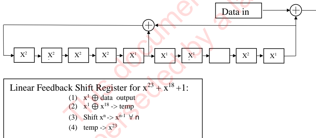
Figure 2-1: Linear Feedback Shift Register
